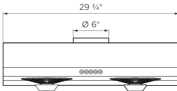
AVANT
