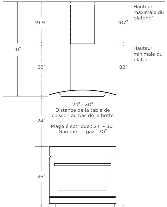
PROLONGEMENT DE LA CHEMINÉE (CHE007, VENDU À PART*)
