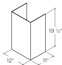
CHEMINÉE INFÉRIEURE
