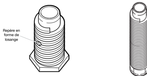
Pied de nivellement avec repère en forme de diamant.
