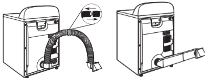
Installation au-dessus de la sécheuse (également offerte avec un coude décalé)
