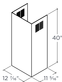
PROLONGEMENT DE LA CHEMINÉE (CHE015, VENDU À PART*)
