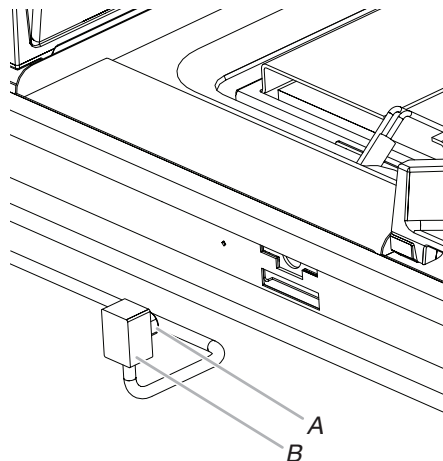
A. Porte-gicteur du grill B. Support de porte-gicteur
