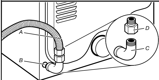
A. Raccord flexible de gaz de 3/8" C. Coude de 3/8" par 3/8" B. Conduit de la sècheuse de 3/8" D. Adaptateur entre le conduit et le joint conique de 3/8"
