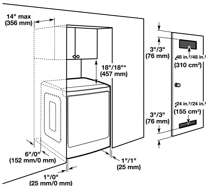
Dégagement minimum/recommandé
