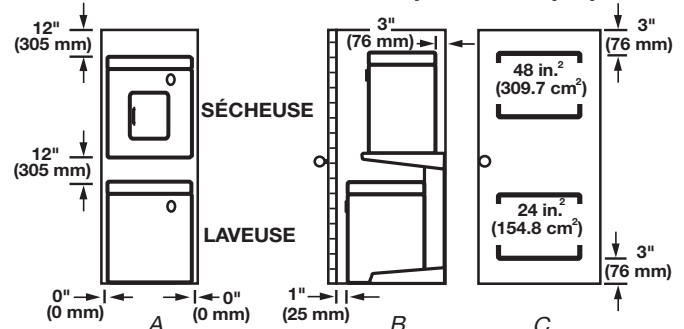
A. Encastrement B. Vue latérale - placard ou endroit exigü C. Porte de placard avec ouvertures d'entrée d'air
