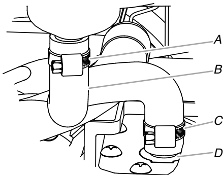
A. Bride de tuyau réglable de \frac{7}{8} " B. Tube de vidange (entre le bac à glaçons et la pompe de vidange)
