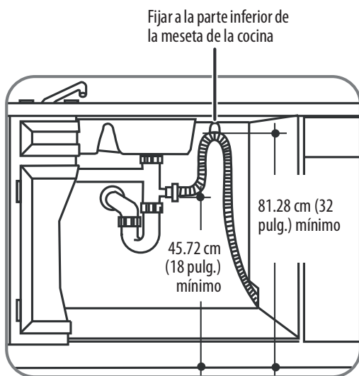
Instalación de la conexión te
