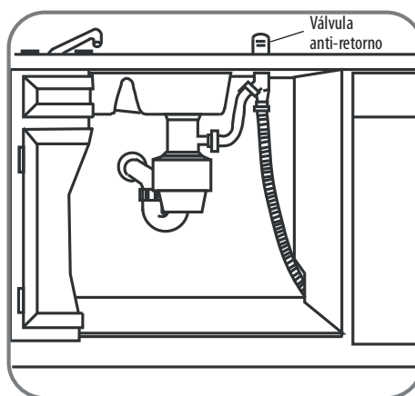
Instalación del triturador de basura
