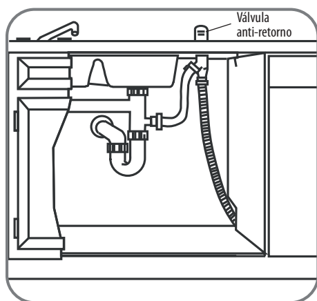
Instalación de la conexión te
