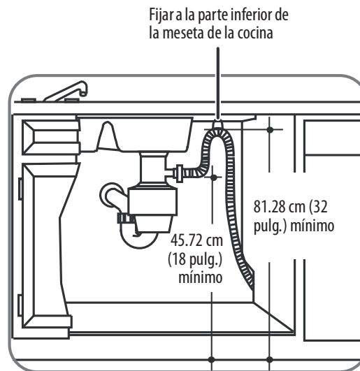
Instalación del triturador de basura
