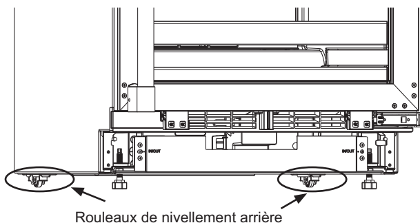
Vis de réglage du rouleau de nivellement arrière
