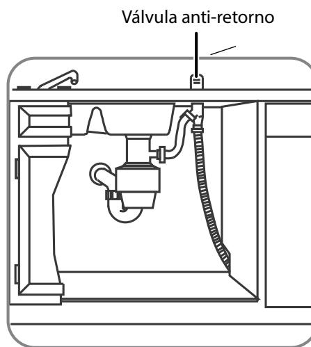
Instalación del triturador de basura
