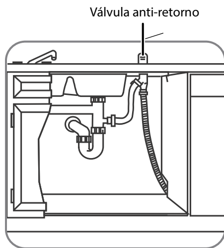
Instalación de la conexión te
