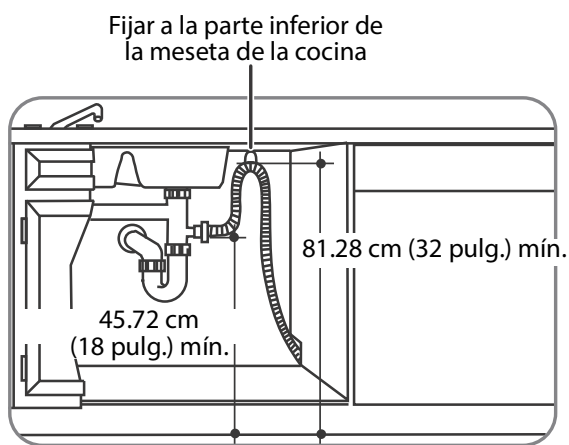
Instalación de la conexión te
