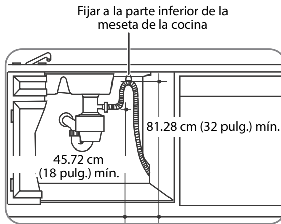
Instalación del triturador de basura
