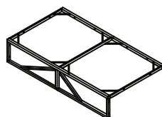
Seat frame of bench /Cadre de siège du banc
