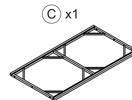
Bench Seat Frame Cadre de la Banquette
