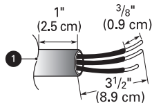
① Placa de conexión del cable/conducto
