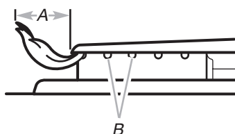
A. 1-1½" (2,5-3,8 cm) B. Orificios del quemador
