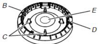
A. Chapeau de brûleur B. Tiges d'alignement C. Allumeur D. Base du brûleur E. Ouverture du tube d'arrivée de gaz
