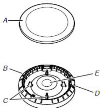
A. Tapa del quemador B. Espigas de alineación C. Encendedor D. Base del quemador E. Apertura del tubo del gas
