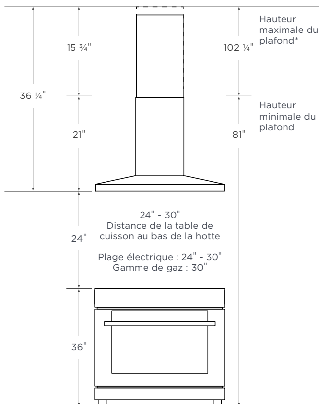
PROLONGEMENT DE LA CHEMINÉE (CHE014, VENDU À PART*)
