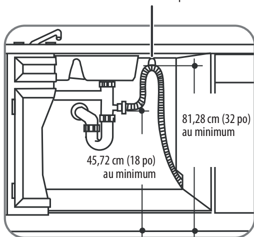
Installation du té de vidange
