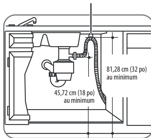
Installation du dispositif d'évacuation de déchets
