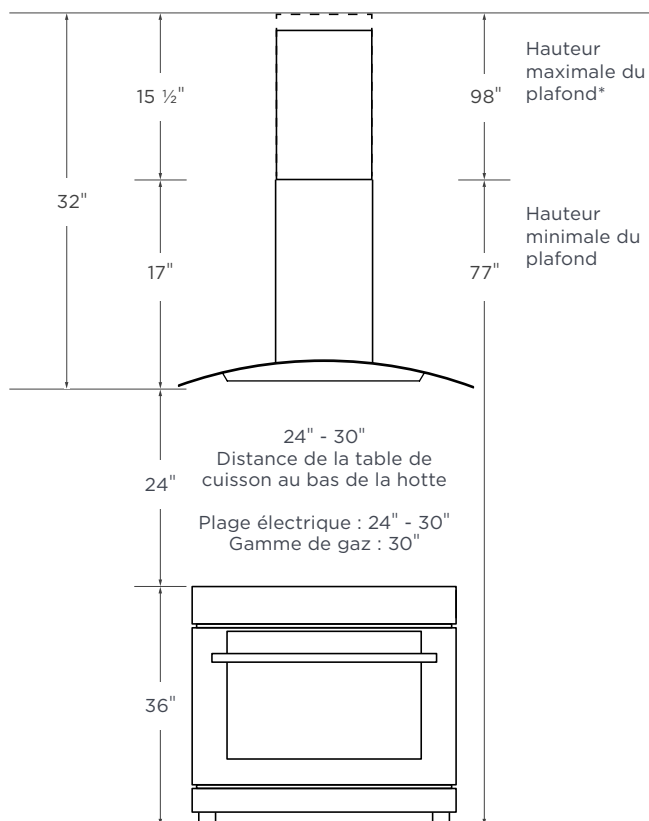
PROLONGEMENT DE LA CHEMINÉE (CHE004, VENDU À PART*)
