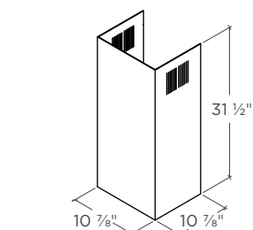
PROLONGEMENT DE LA CHEMINÉE (CHE004, VENDU À PART*)
