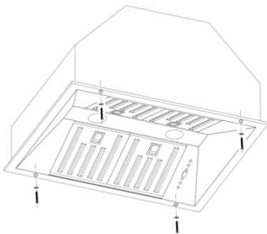
FRHRE5337-30 : 4 vis.
