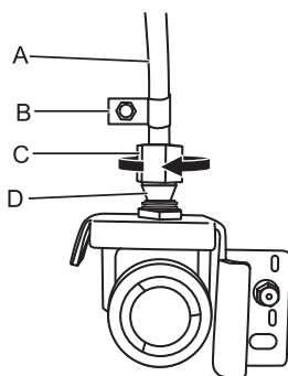
A. Tuyau en cuivre ou en polyéthylène réticulé B. Collier en « P » C. Écrou de compression D. Virole de compression
