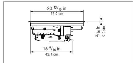
Fig. 5.6 Dimensiones del aparato vista lateral
