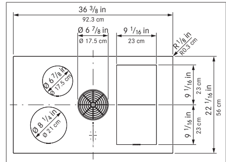
Fig. 5.4 Dimensiones del aparato vista superior
