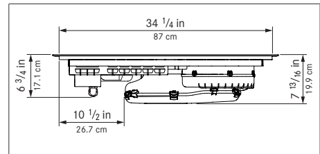
Fig. 5.5 Dimensiones del aparato vista frontal
