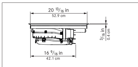
Fig. 5.6 Vue latérale
