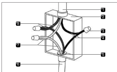
Fig. 11.21 Câble 3 fils
