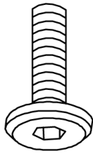
ALLEN KEY SCREW M6 X 30 mm QTY 1
