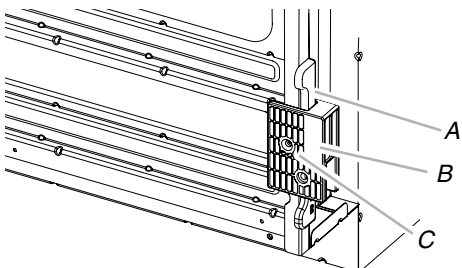
A. Spacer B. Foot C. #8-18 x 3/8" screw
