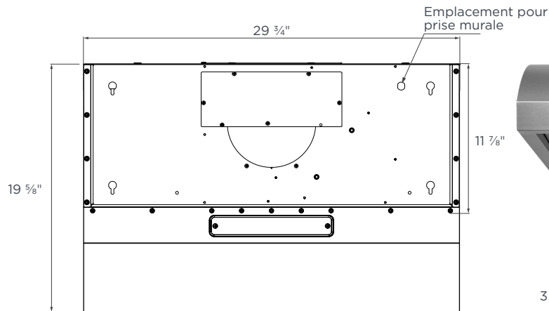
DESSUS
