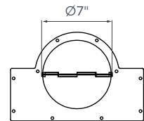
ADAPTATEUR D'ÉCHAPPEMENT ROND
