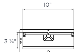
ADAPTATEUR D'ÉCHAPPEMENT RECTANGULAIRE SUPÉRIEUR / ARRIÈRE
