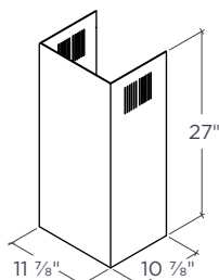
PROLONGEMENT DE LA CHEMINÉE (CHE007, VENDU À PART*)
