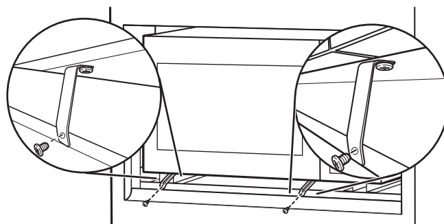
Supports de fixation du conduit inférieur
