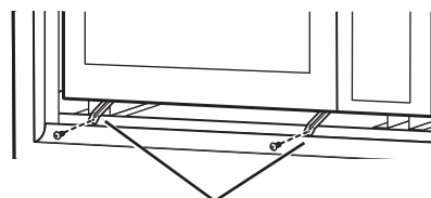
Supports de fixation du conduit inférieur
