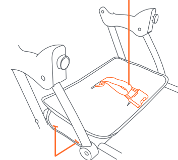
Button pad to stroller Abroche la almohadilla al carrito Boutonnez la garniture à la poussette
