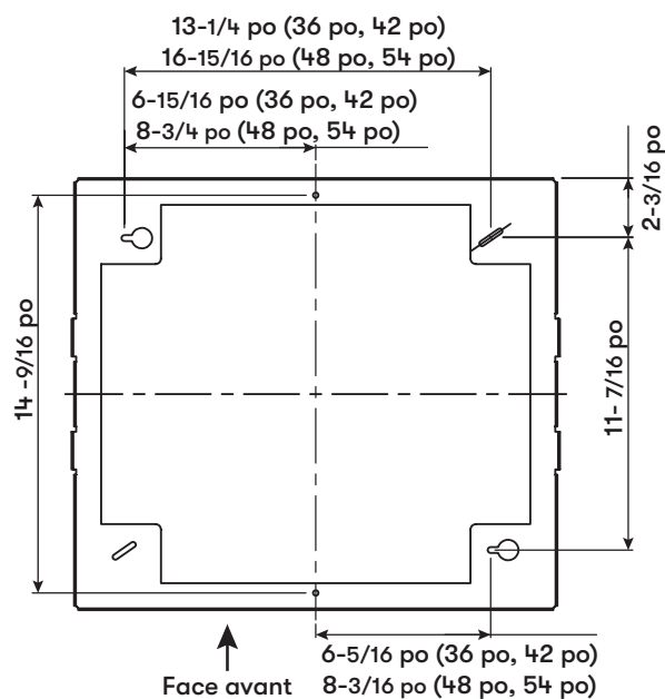
CADRE DE SUPPORT SUPÉRIEUR (vue de dessus)
