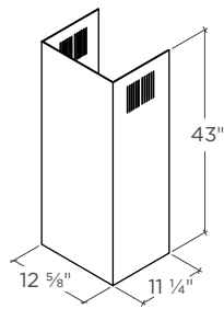
PROLONGEMENT DE LA CHEMINÉE (CHE014, VENDU À PART*)
