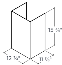
CHEMINÉE INFÉRIEURE
