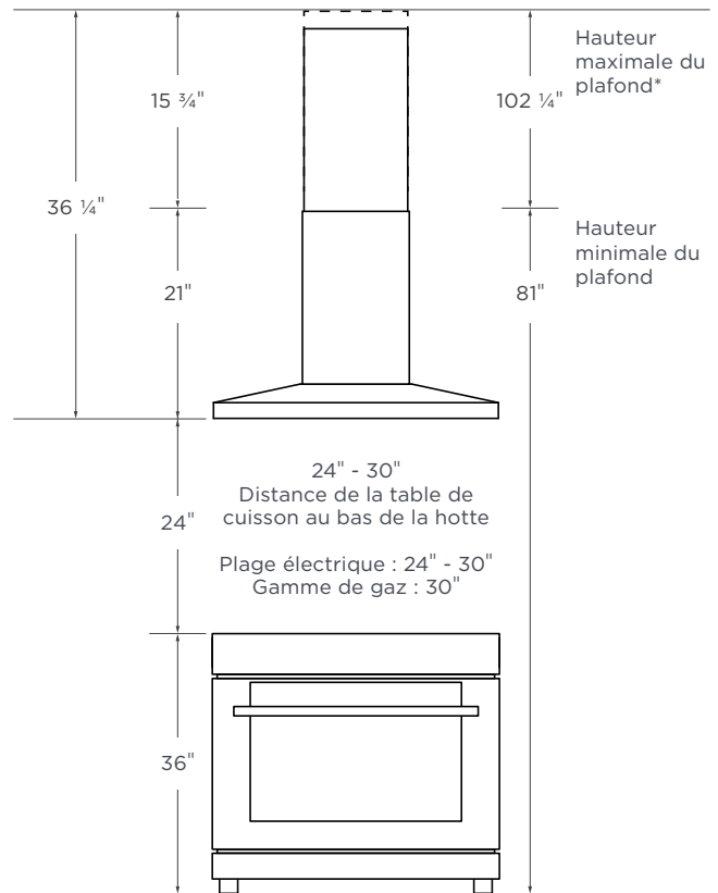
PROLONGEMENT DE LA CHEMINÉE (CHE014, VENDU À PART*)
