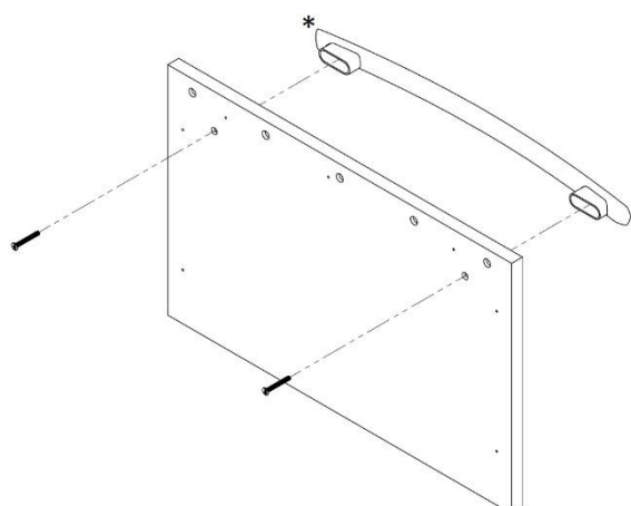
Tornillo plano al ras de la superficie (Fig. A)
