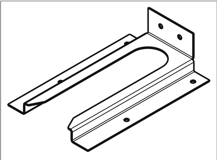
Figura 7: Soporte antivuelco
