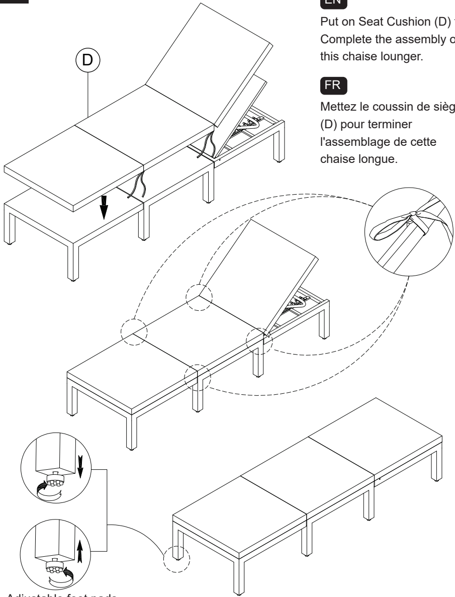
Adjustable feet pads /Patins réglables pour les pieds
