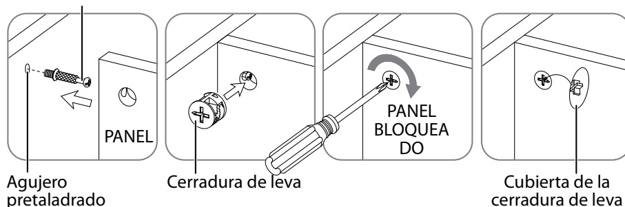
Pasador de leva
