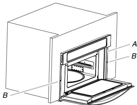
A. Glissière de montage
