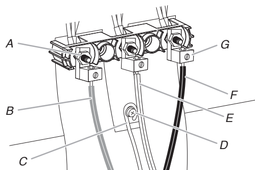
A. Tuerca hexagonal 10-32 B. Línea 2 (roja) C. Hilo desnudo de conexión a tierra (verde) D. Tornillo de puesta a tierra E. Hilo neutro (blanco) F. Línea 1 (negra) G. Lengüeta de terminal
