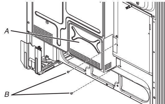
A. Tapa del bloque de terminal B. Tornillos (2)
