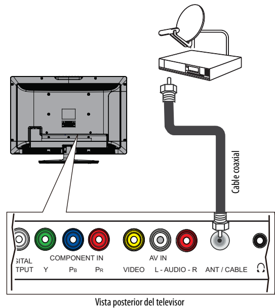
Decodificador de cable o receptor de satélite
