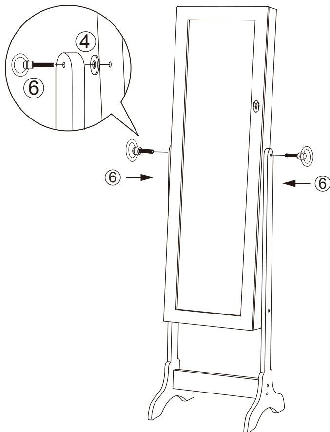
SPACER /RONDELLE
