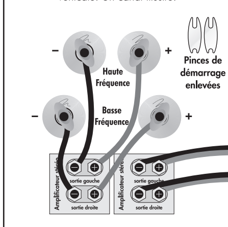
Fig. 4: Raccordement par bi-amplification verticale. Un canal illustré.
