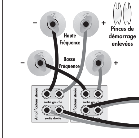
Fig. 3: Raccordement par bi-amplification horizontale. Un canal illustré.
