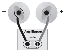
Fig. 1a: Raccord à un fil. Un canal illustré.
