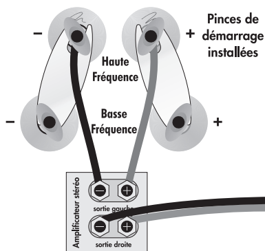
Fig. 1b: Raccord à un fil. Un canal illustré.
