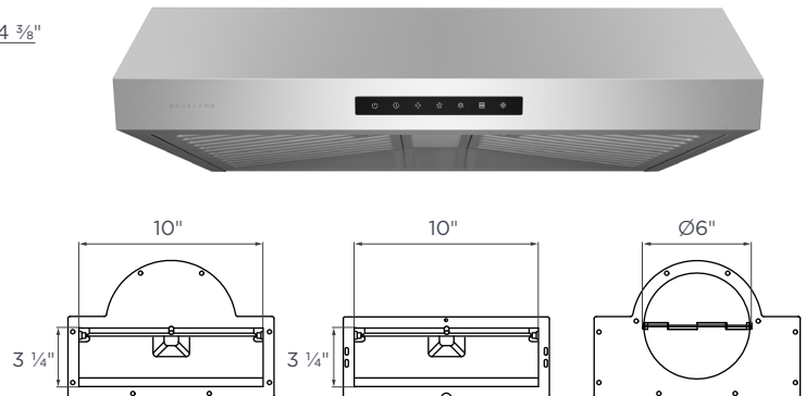
ADAPTATEUR D'ÉCHAPPEMENT RECTANGULAIRE SUPÉRIEUR
