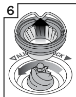
Retirer la meule supérieure
