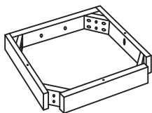
Seat Frame /Cadre du Siège
