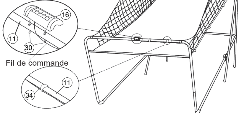
FIG.11A Boîtier de commande
