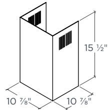
CHEMINÉE SUPÉRIEURE
