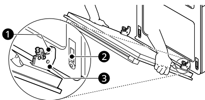
1 Brazo de la bisagra 2 Borde inferior de la ranura 3 Hendidura
