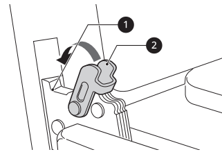
1 Brazo de la bisagra 2 Traba de la bisagra
