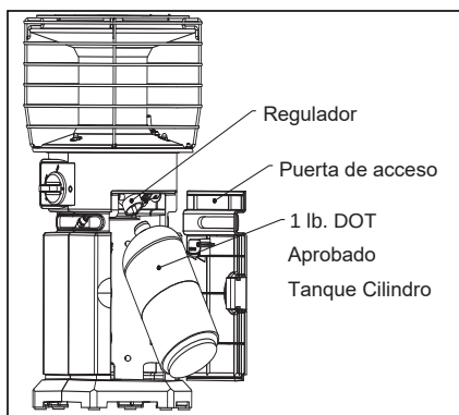
Fig. 1 - Instalación del tanque del cilindro de 1 lb
