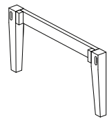
Chair side frame without hole /Cadre latéral de la chaise sans trou B x 7
