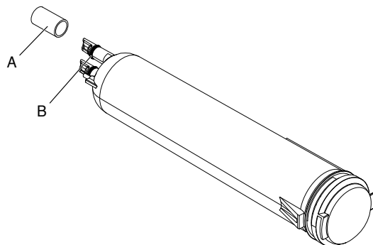
A. Cubierta B. Juntas tóricas
