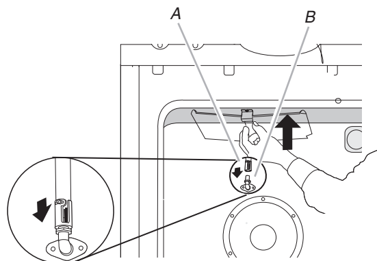
A. Gicleur de brûleur de grill
