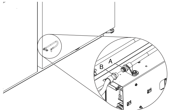
A. Point d'entrée du raccordement à l'alimentation en eau
