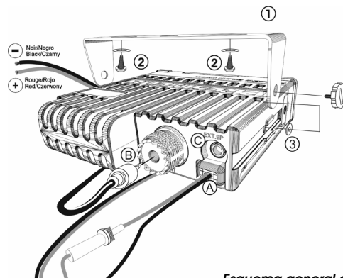
Esquema general de montaje
